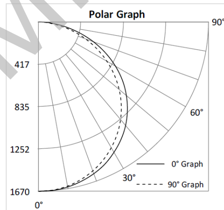
PLX-SEL-24-50L Luminaire Data
